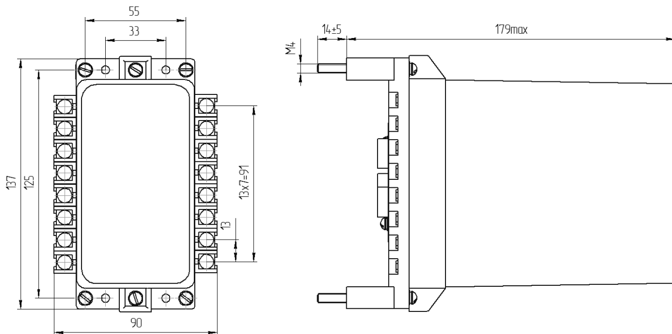
Переднее присоединение РСТ-40ВО
